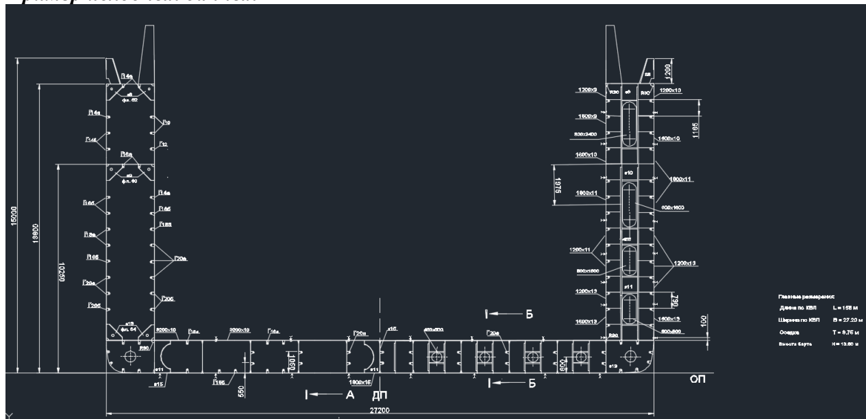
Рисунок 1 – Чертеж мидель-шпангоута
